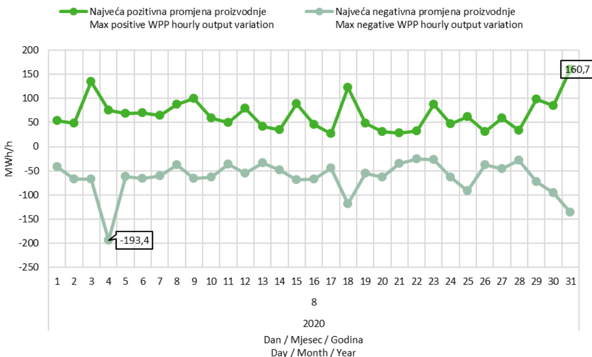
Slika 9 Maksimalna pozitivna i maksimalna negativna promjena satne proizvodnje VE u kolovozu 2020. godine
