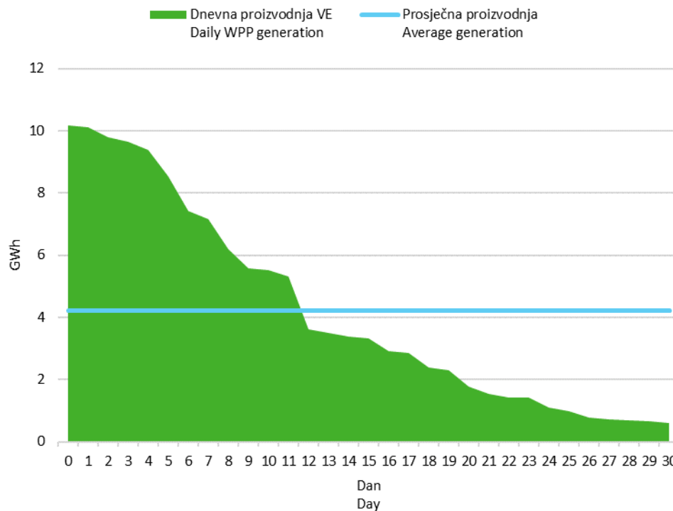
Slika 6 Krivulja trajanja dnevne proizvodnje vjetroelektrana u kolovozu 2020. godine
