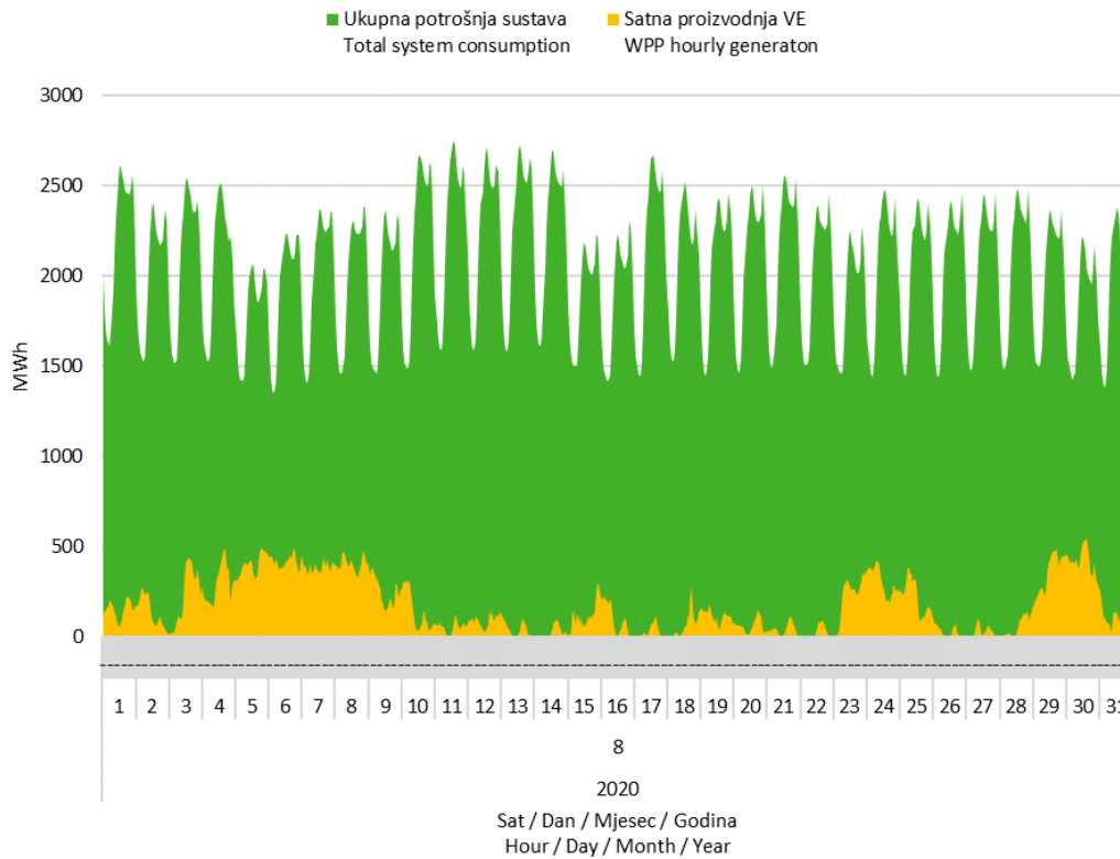
Slika 7 Usporedba satnog dijagrama opterećenja sustava i proizvodnje vjetroelektrana u kolovozu 2020. godine
