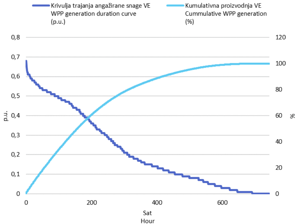
Slika 3 Krivulja trajanja angažirane snage svih VE i kumulativna proizvodnja VE u kolovozu 2020. godine u jediničnim vrijednostima
