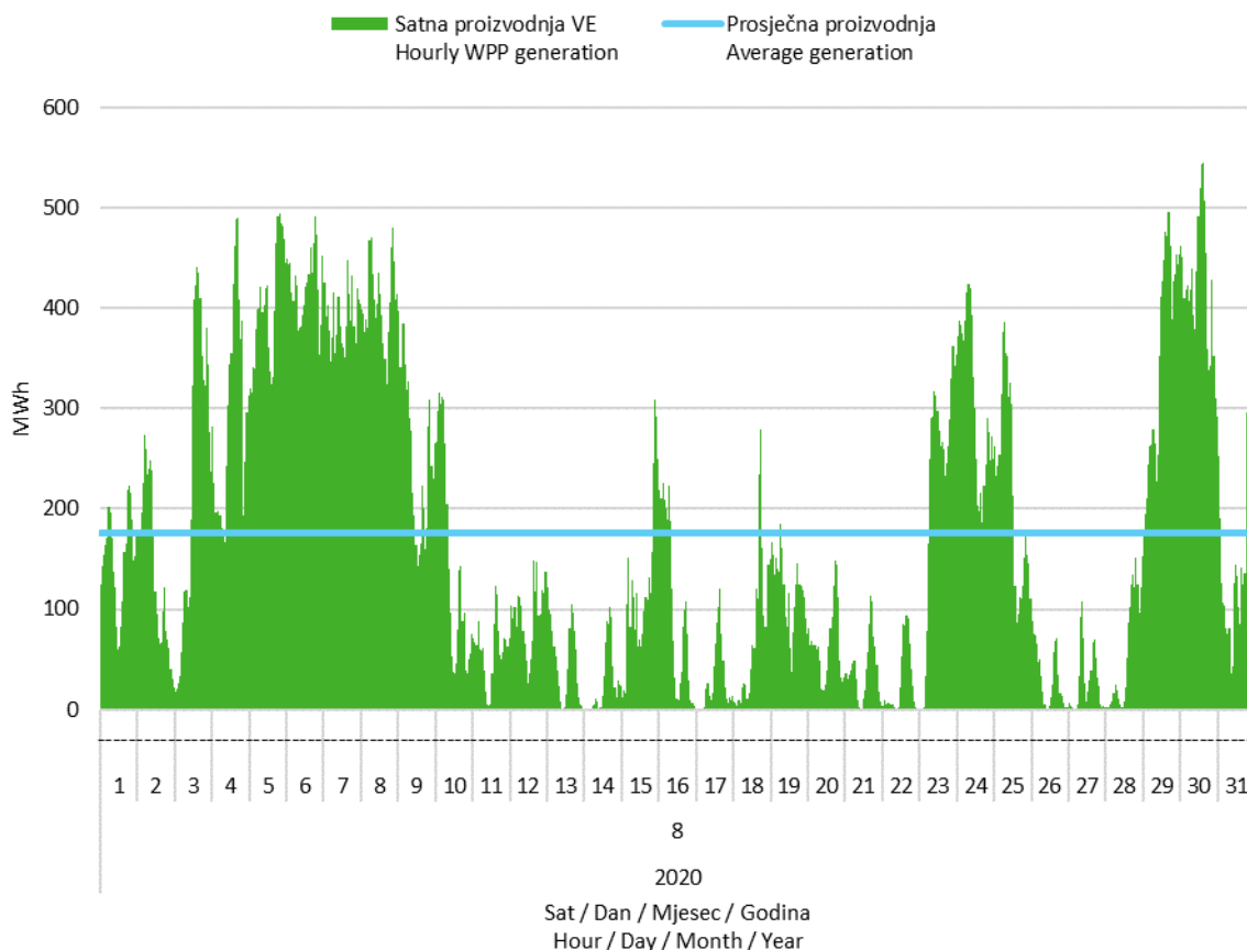
Slika 2 Satna proizvodnja svih vjetroelektrana u kolovozu 2020. godine
