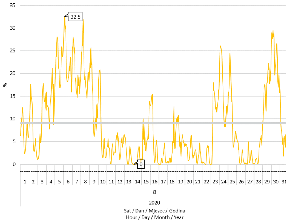
Slika 8 Udio proizvodnje vjetroelektrana u pokrivanju satnog opterećenja elektroenergetskog sustava u kolovozu 2020. godine
