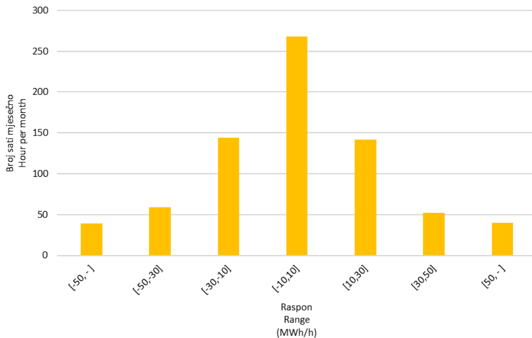
Slika 10 Statistička raspodjela satnih promjena proizvodnje VE u kolovozu 2020. godine
