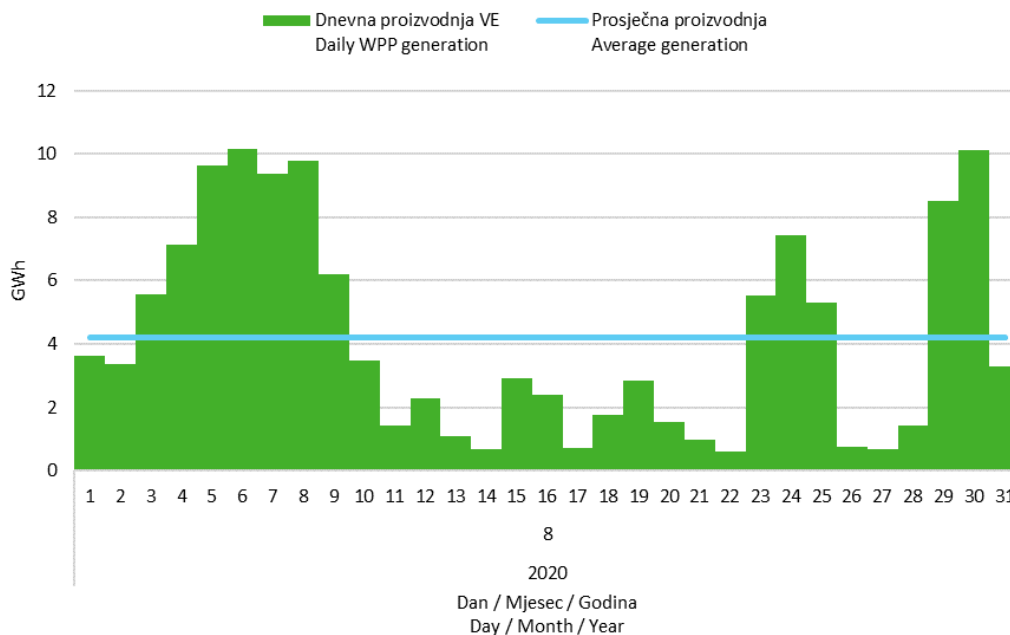
Slika 5 Dnevna proizvodnja svih vjetroelektrana u kolovozu 2020. godine
